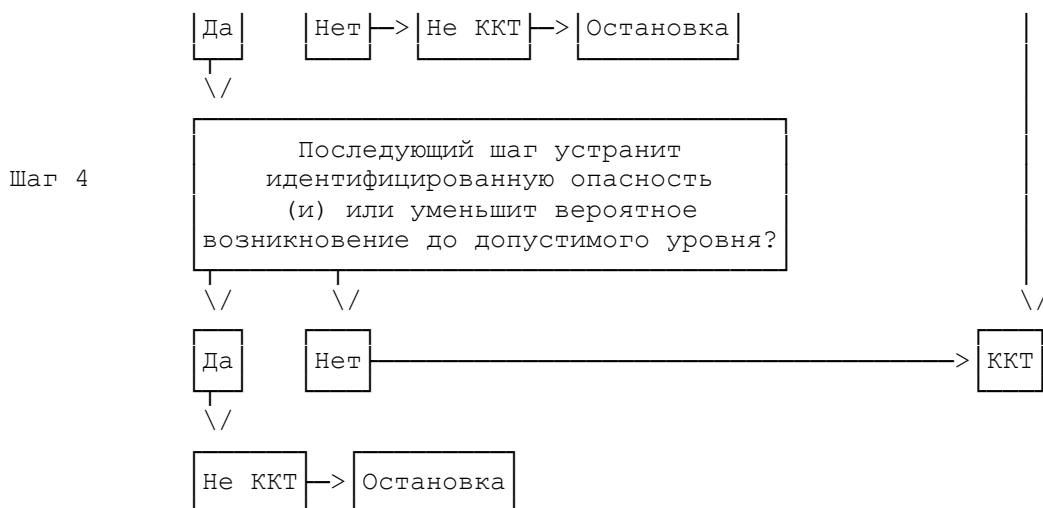
Рисунок В.1 - Пример дерева решений, идентифицирующего критические контрольные точки
